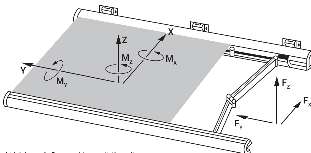
Abbildung 4: Systemskizze mit Koordinatensystem
