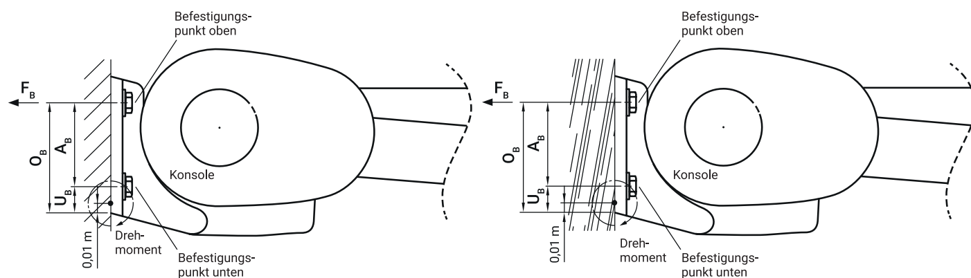
Abbildung 7: Lastenleitung an der Konsole mit druckfestem Untergrund
