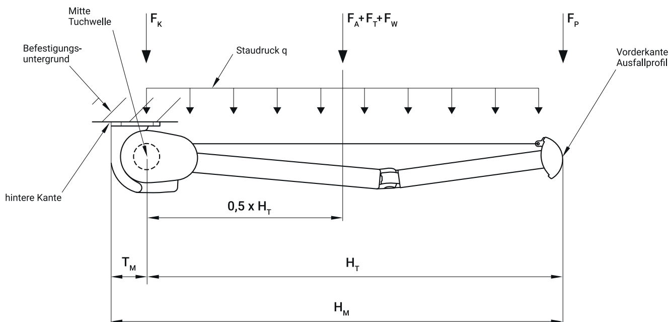
Abbildung 14: Statisches System mit Lastangriffspunkten
