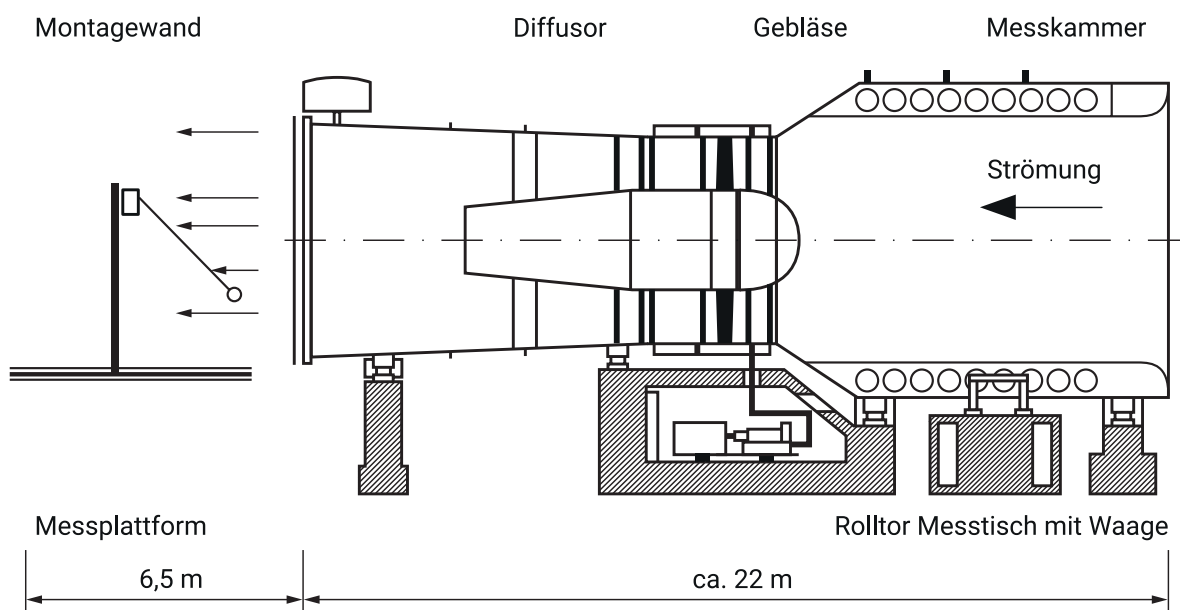
Abbildung 2: Aufbau des Windkanals und der entsprechenden Prüfeinrichtungen
