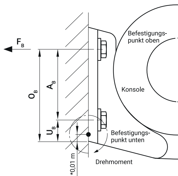
Abbildung 25: Lastenleitung an der Konsole
