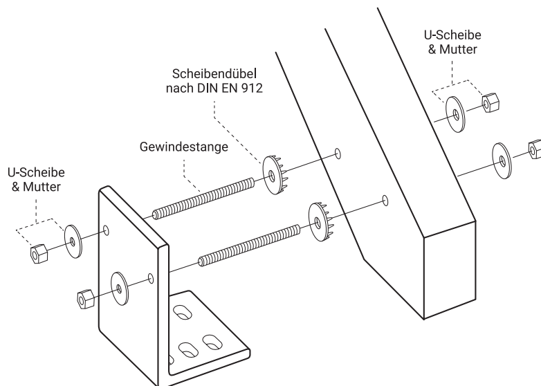
Abbildung 23: Einseitige Dachsparrenkonsole
