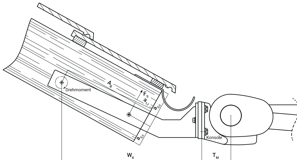
Abbildung 39: Lasteinleitung an der Konsole
