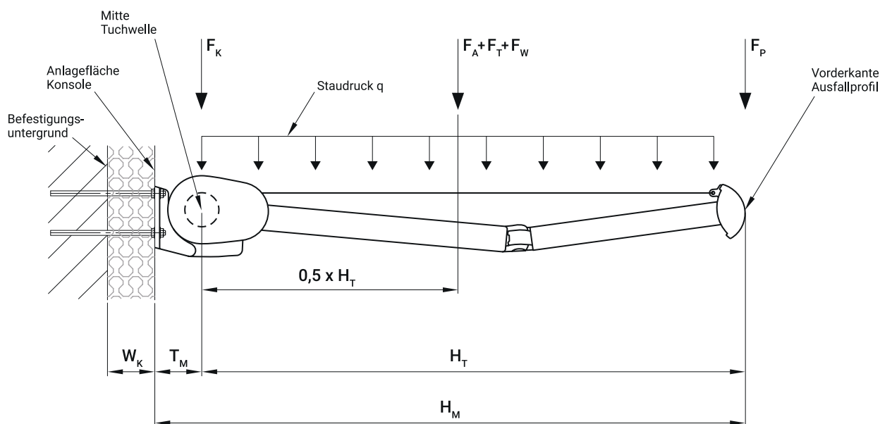
Abbildung 26: Statisches System mit Lastangriffspunkten
