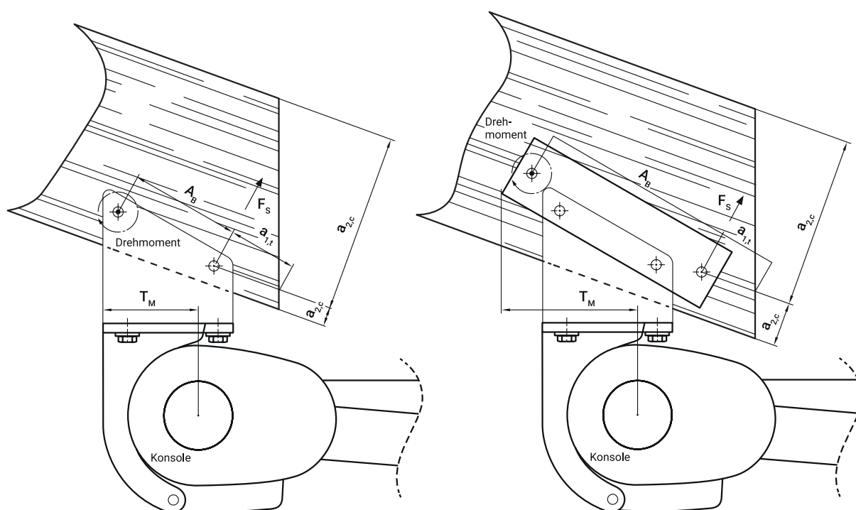
Abbildung 17: Lastenleitung an der Markisenbefestigung auf Holz (Dachsparrenbefestigung)
