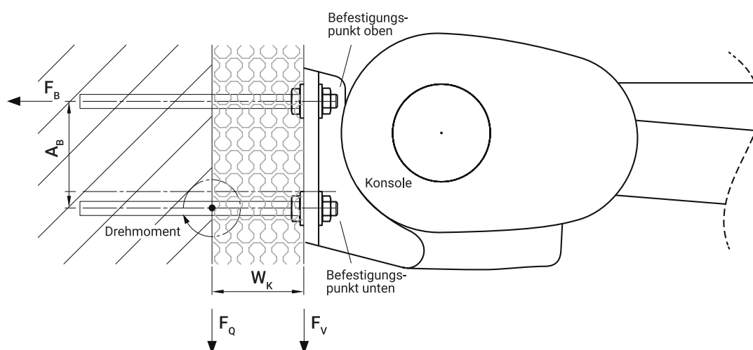
Abbildung 9: Lastenleitung an der Konsole mit nicht-druckfestem Untergrund
