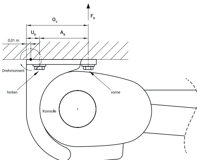
Abbildung 33: Lasteinleitung an der Konsole
