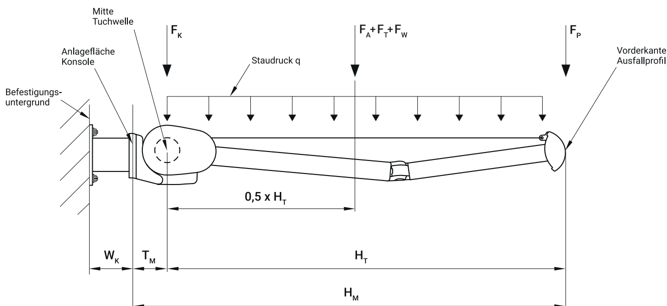
Abbildung 10: Statisches System mit Lastangriffspunkten
