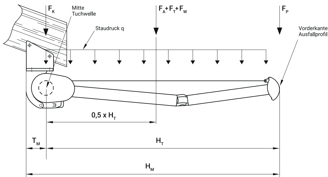
Abbildung 34: Statisches System mit Lastangriffspunkten
