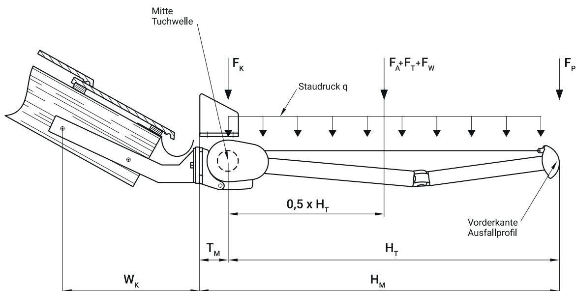
Abbildung 18: Statisches System mit Lastangriffspunkten
