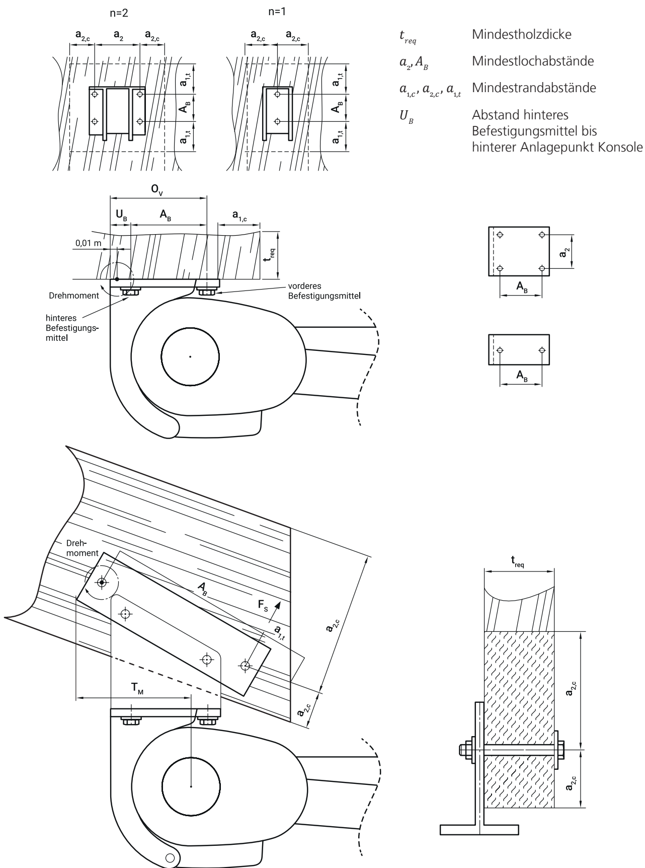
Abbildung 21: Randabstände bei Befestigung auf Holz
