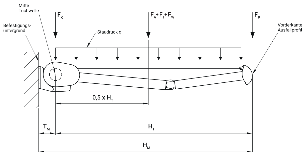
Abbildung 6: Statisches System mit Lastangriffspunkten
