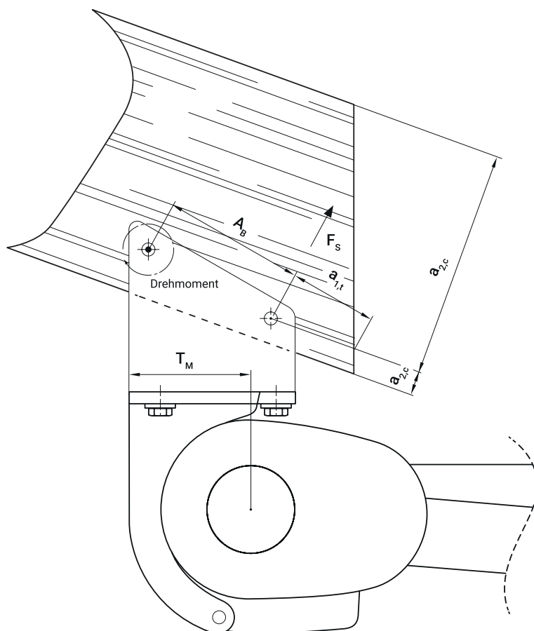
Abbildung 36: Lasteinleitung an der Konsole
