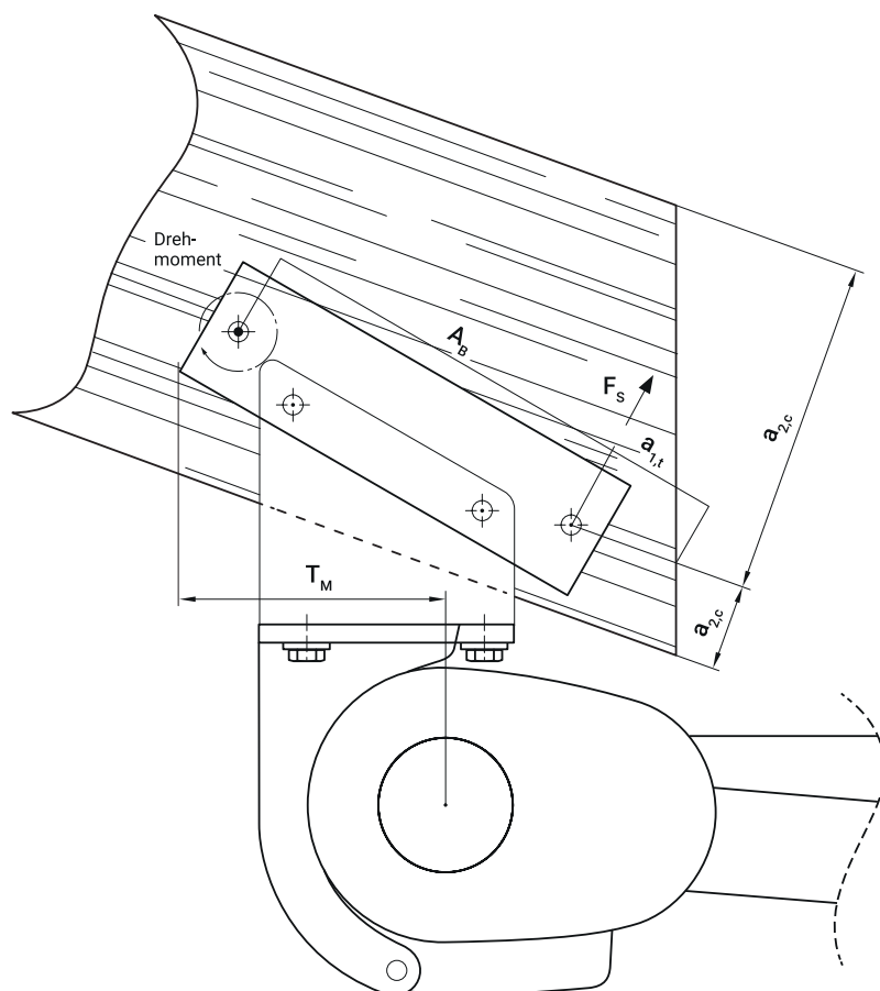
Abbildung 37: Lasteinleitung an der Konsole
