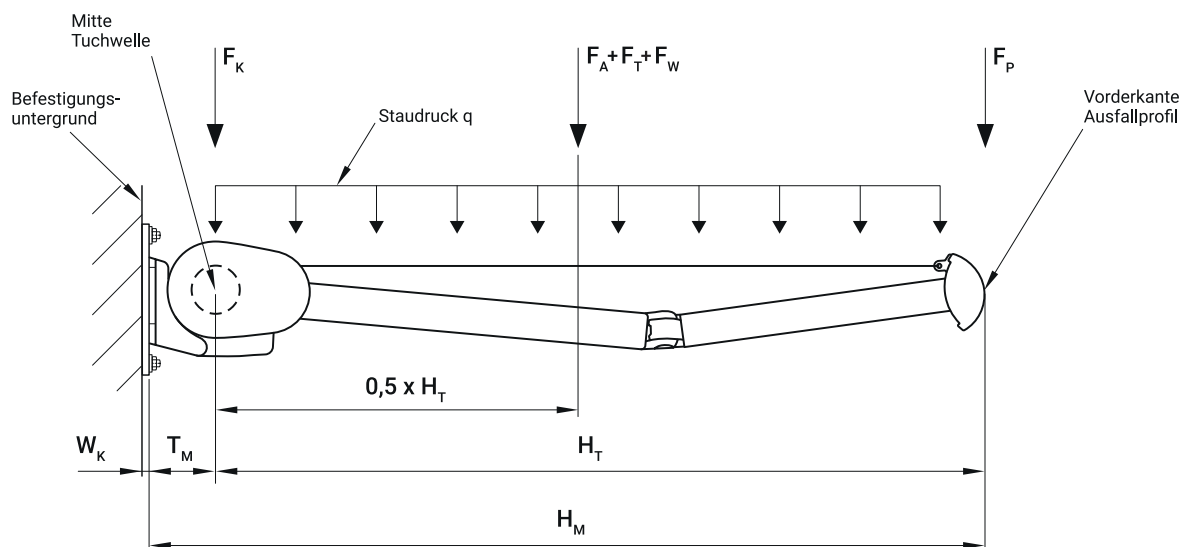
Abbildung 30: Statisches System mit Lastangriffspunkten
