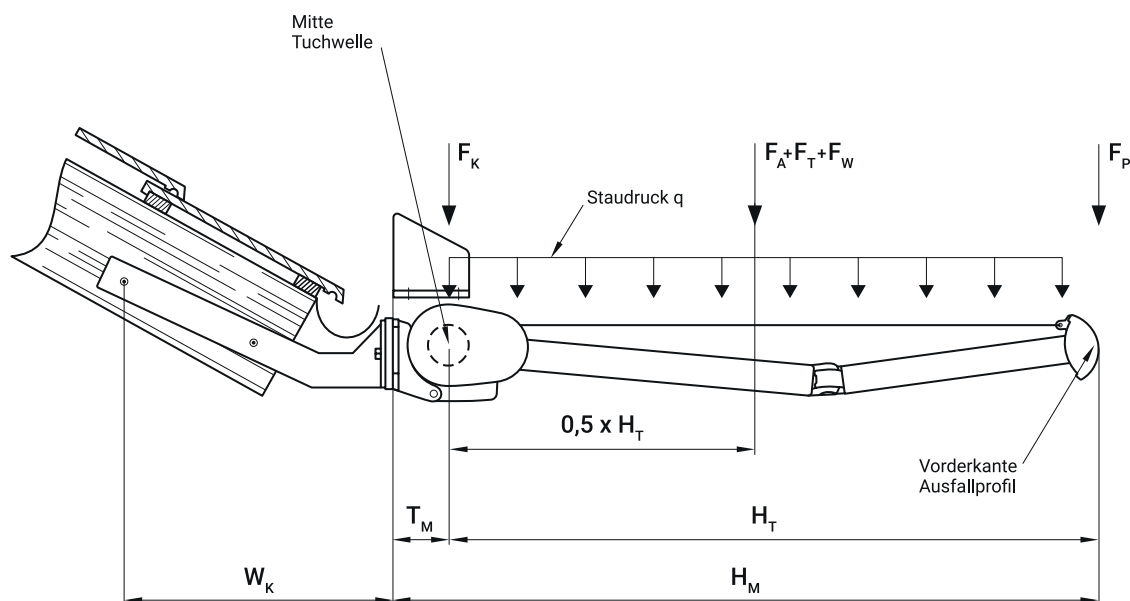
Abbildung 38: Statisches System mit Lastangriffspunkten
