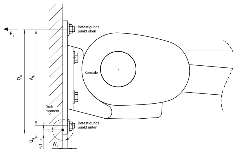
Abbildung 31: Lastenleitung an der Konsole
