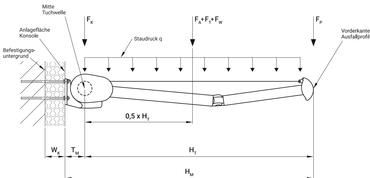
Abbildung 8: Statisches System mit Lastangriffspunkten
