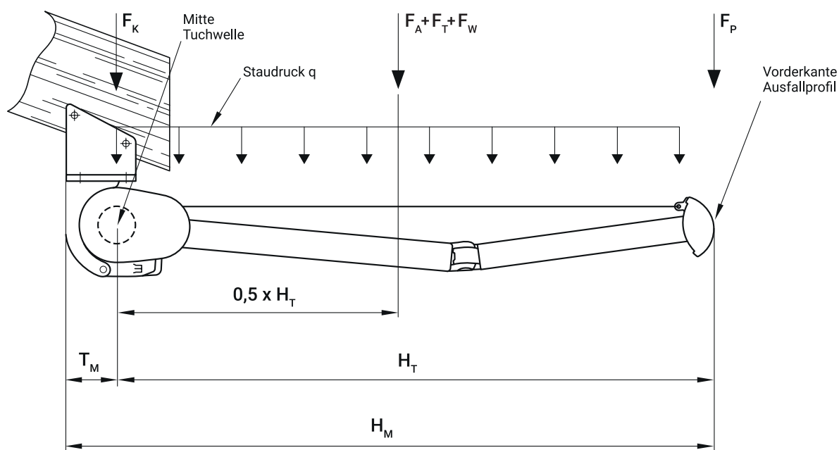
Abbildung 16: Statisches System mit Lastangriffspunkten
