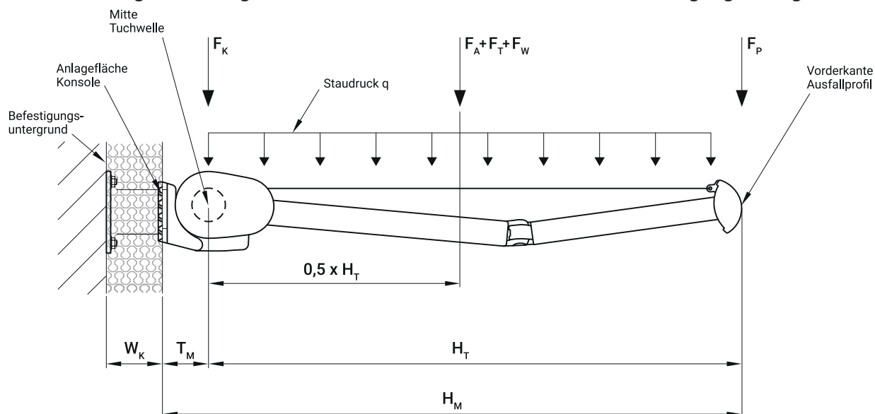
Abbildung 28: Statisches System mit Lastangriffspunkten
