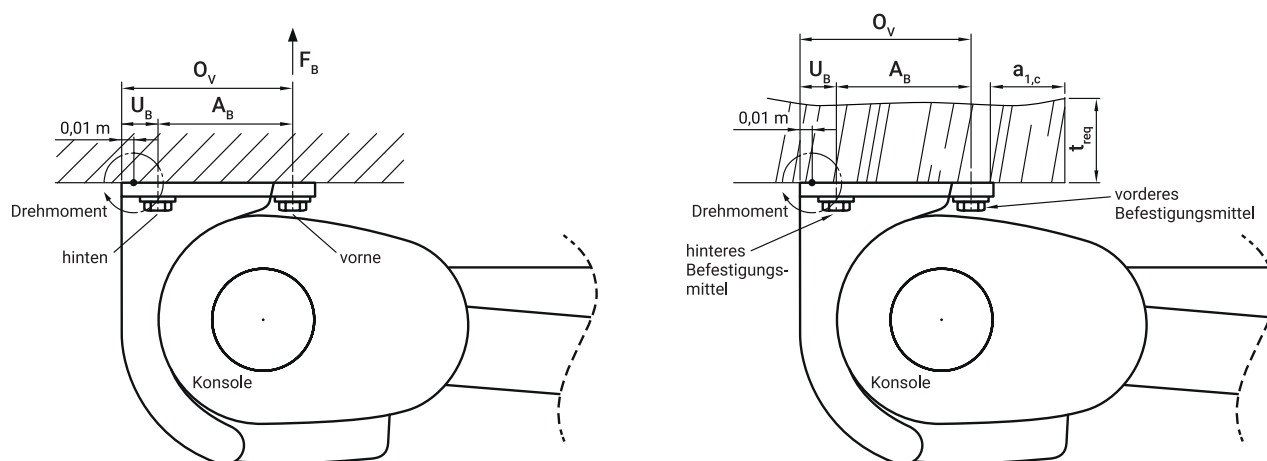
Abbildung 15: Lastenleitung an der Markisenbefestigung mit Deckenhalter der Konsole
