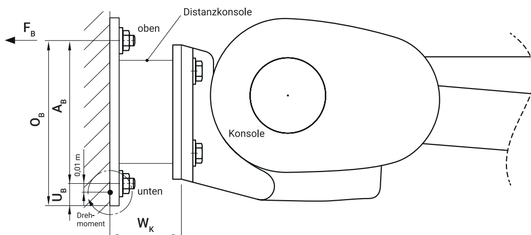
Abbildung 11: Lastenleitung an der Konsole mit Distanzhalter
