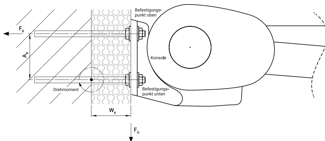
Abbildung 27: Lastenleitung an der Konsole
