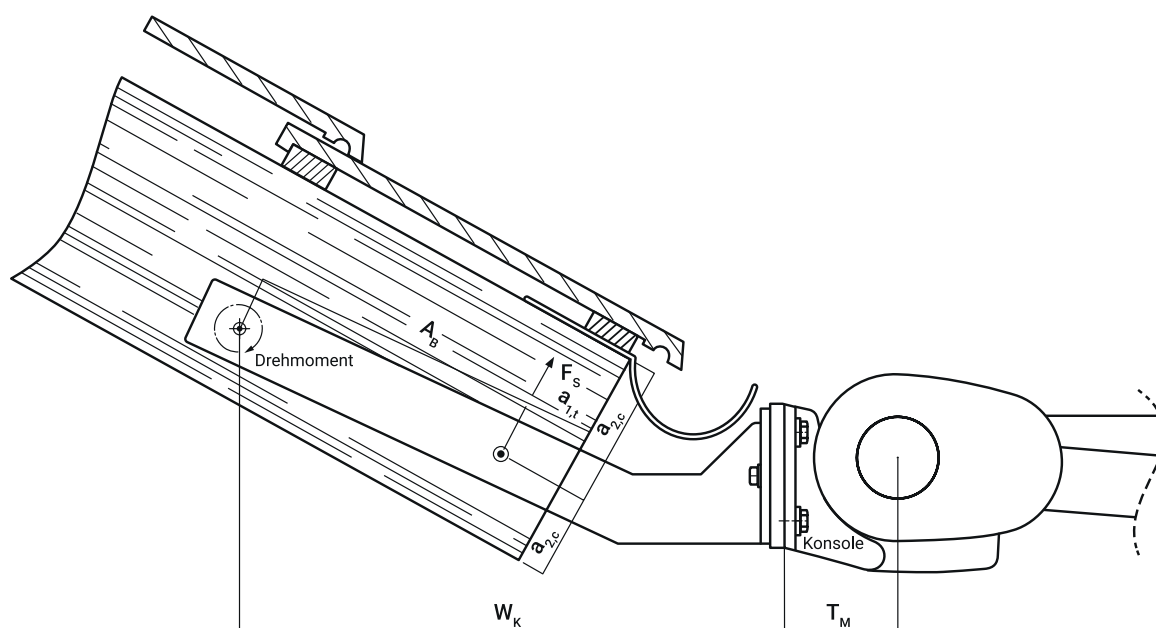
Abbildung 19: Lastenleitung an der Markisenbefestigung auf Holz (Dachsparrenbefestigung)
