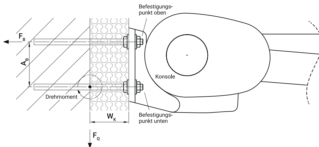
Abbildung 20: Lastenleitung der Querlast an der Konsole
