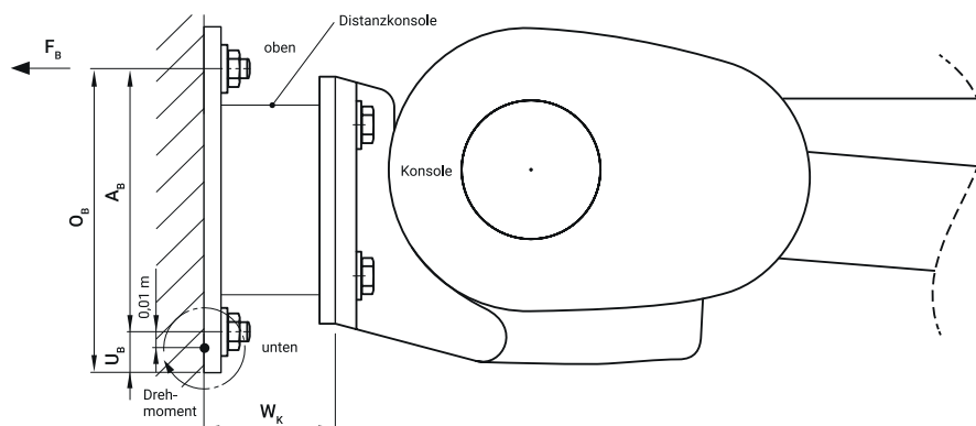
Abbildung 29: Lastenleitung an der Konsole
