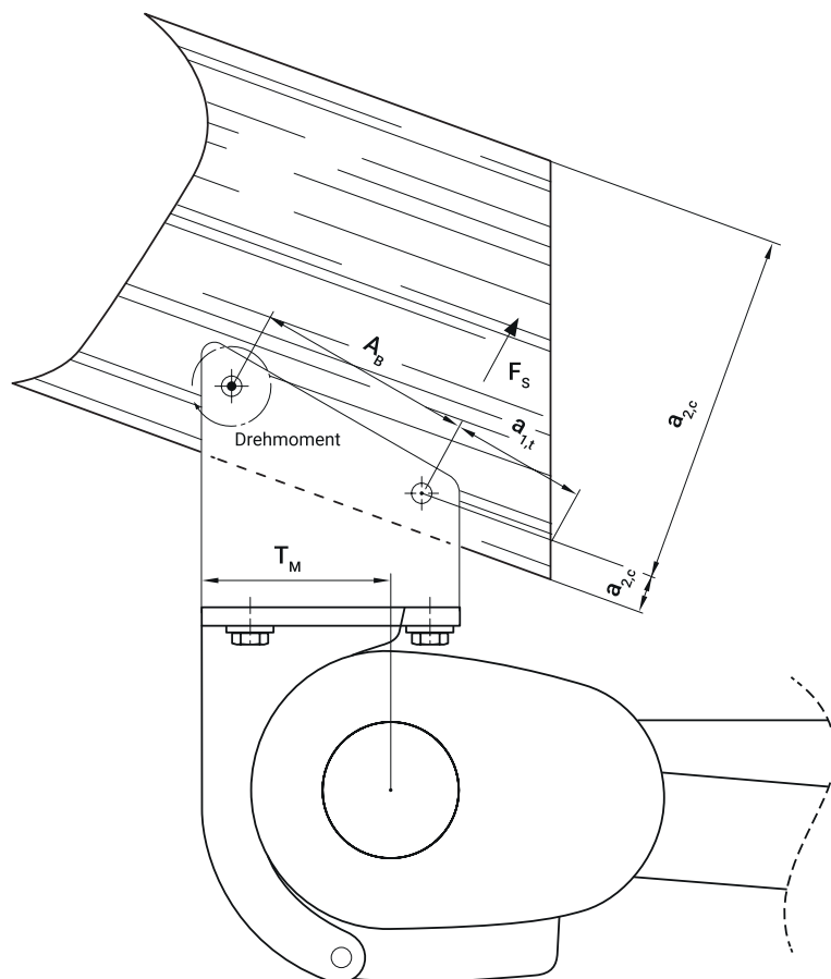
Abbildung 35: Lastenleitung an der Konsole
