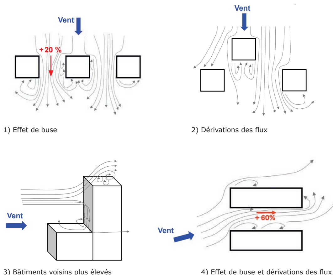
Fig. 6.3 : illustration simplifiée du flux autour d'un bâtiment, y compris les bâtiments environnants
