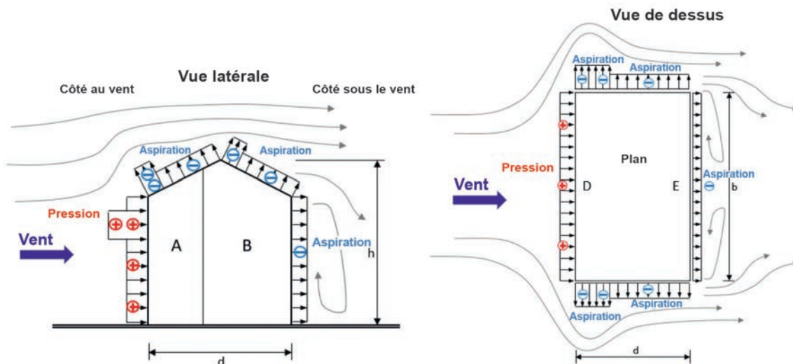
Fig. 6.2 : Illustration simplifiée du flux autour d'un bâtiment indépendant en vue latérale (à gauche) et en vue de dessus (à droite) avec les zones de pression et d'aspiration sur les surfaces du toit et de la façade
