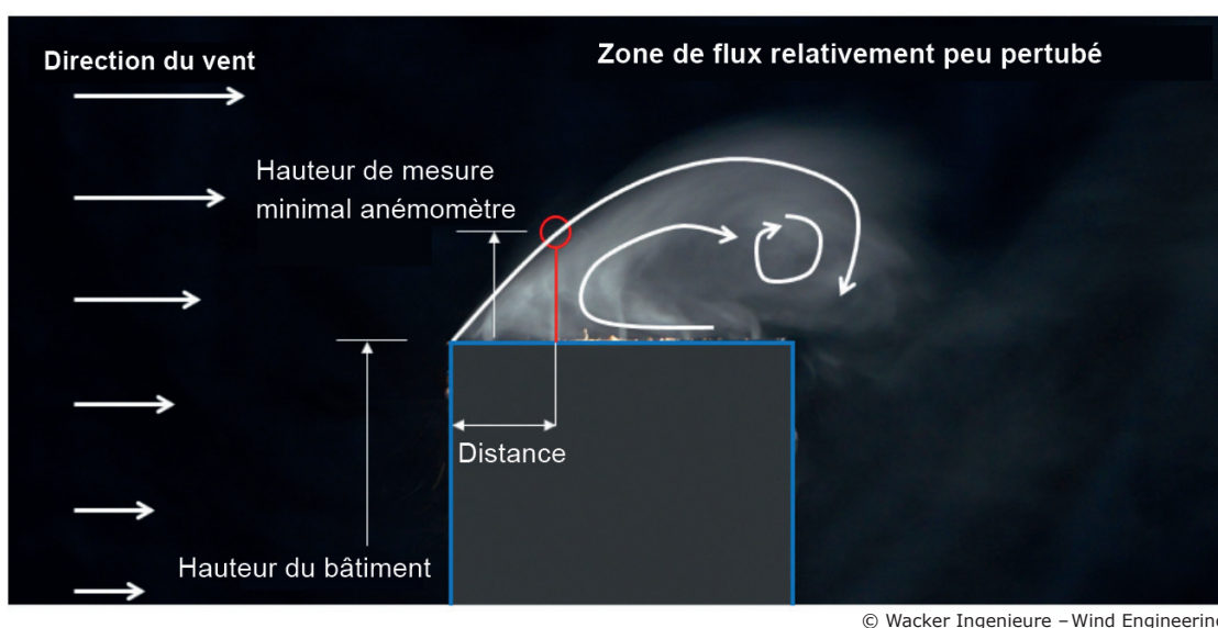
Fig. 6.5 : Visualisation du flux d'air sur un bâtiment dans la soufflerie avec la hauteur de mesure requise d'un anémomètre monté sur le toit
