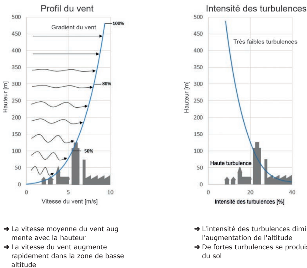
Fig. 6 : trajectoire qualitative, en fonction de la hauteur, de la vitesse moyenne du vent (à gauche) et de l'intensité de la turbulence (à droite) du flux d'une couche limite atmosphérique
