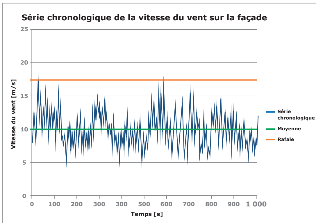
Fig. 6.4 : Représentation d'un exemple de signal de mesure de la vitesse du vent sur la façade du bâtiment
